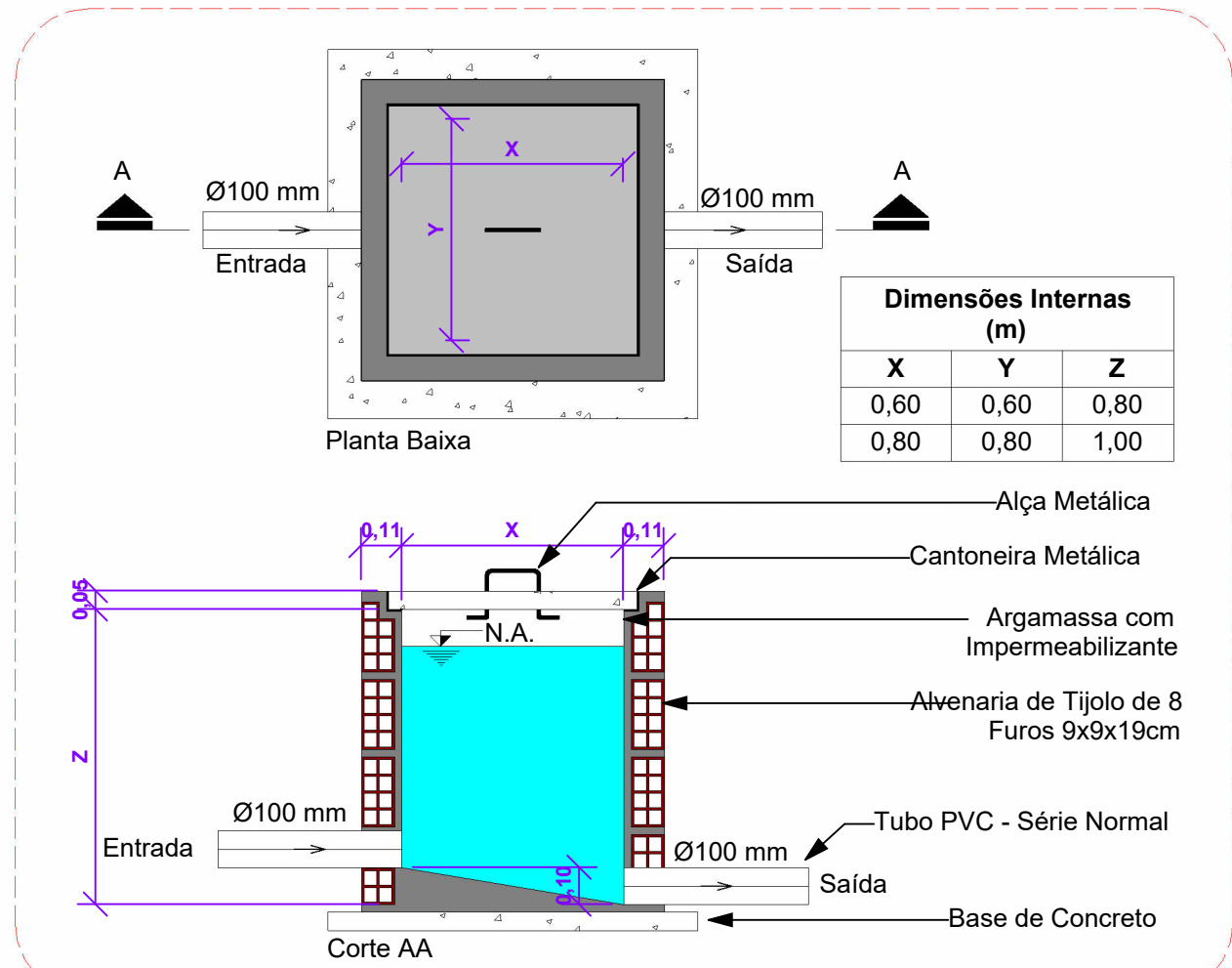
08 - Detalhe - Caixa de Inspeção 1 : 20
