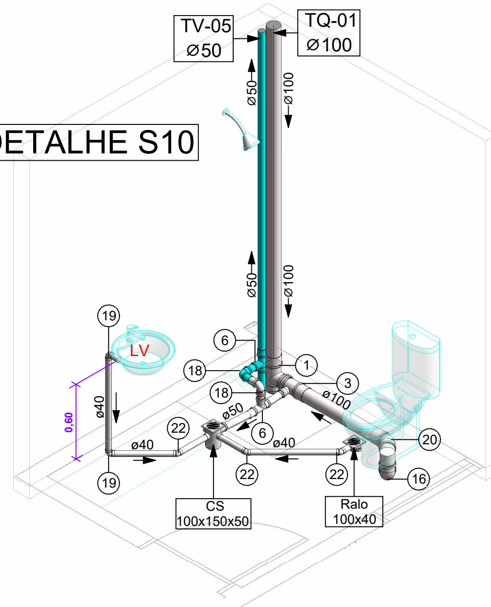
ISO DETALHE S10
