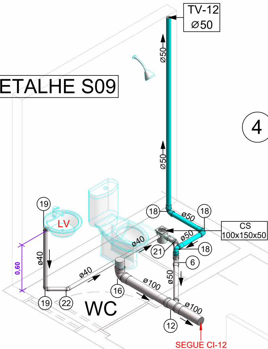
ISO DETALHE S09
