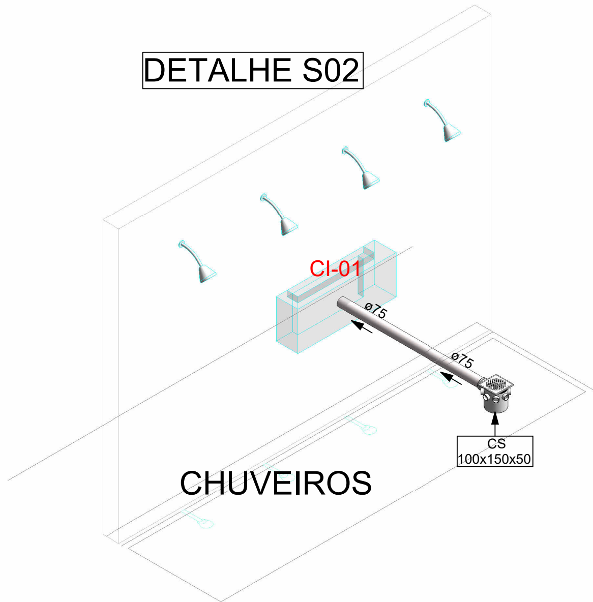
ISO DETALHE S02
