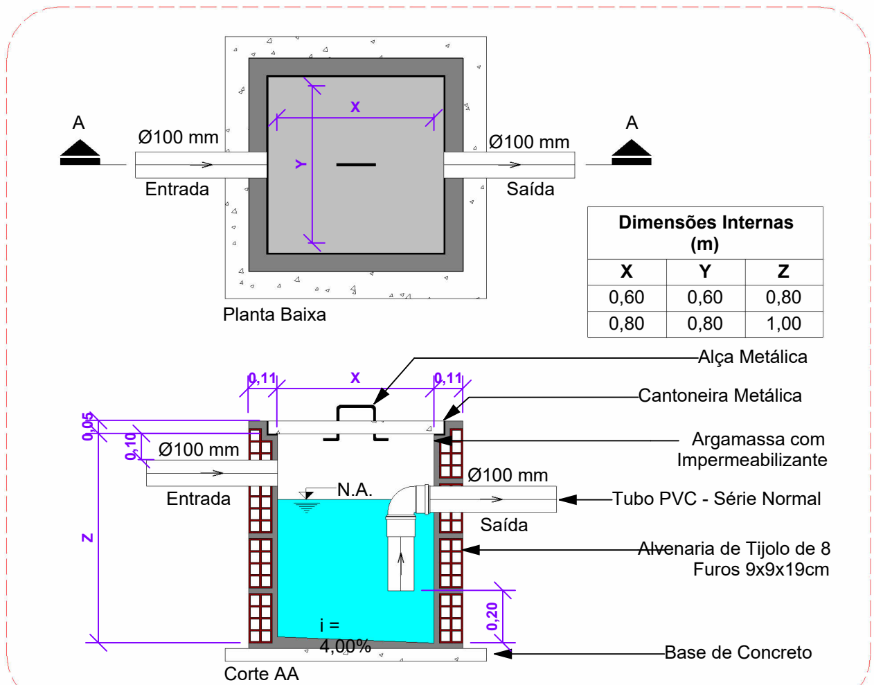
09 - Detalhe - Caixa Sifonada 1 : 20
