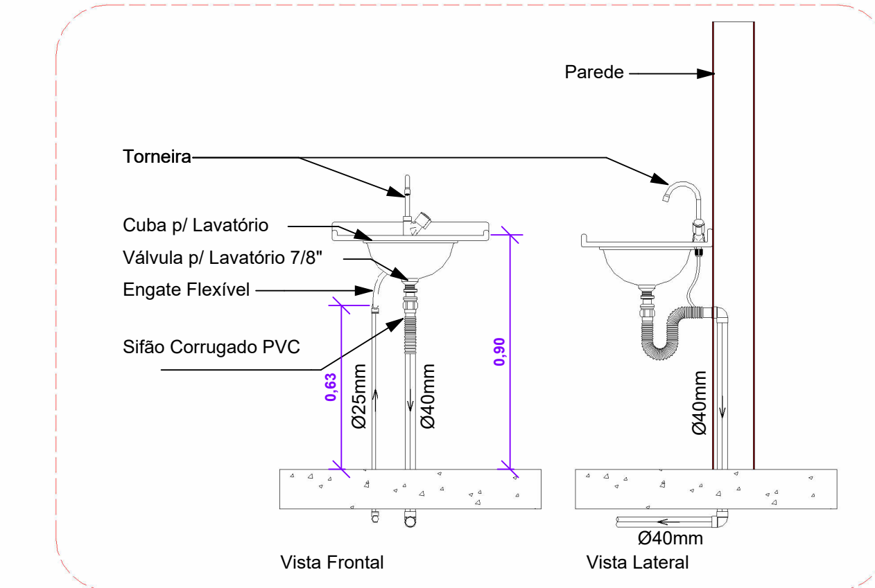
10 - Detalhe - Lavatório 1 : 20
