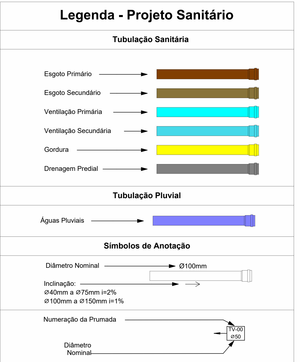
05 - Legenda - Tubulação Sanitária 1 : 20
