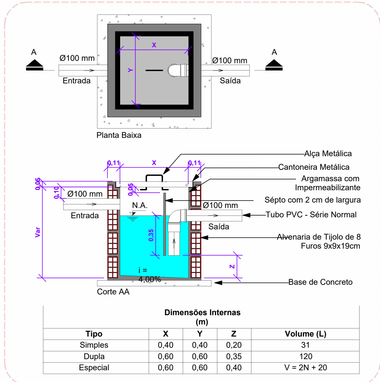
07 - Detalhe - Caixa de Gordura 1 : 20
