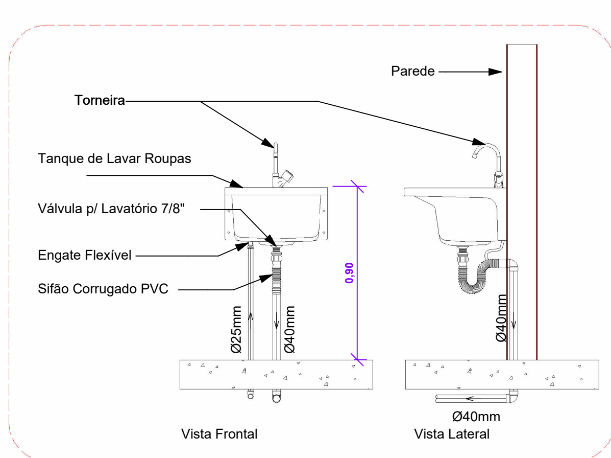
13 - Detalhe - Tanque de Lavar Roupas 1 : 20
