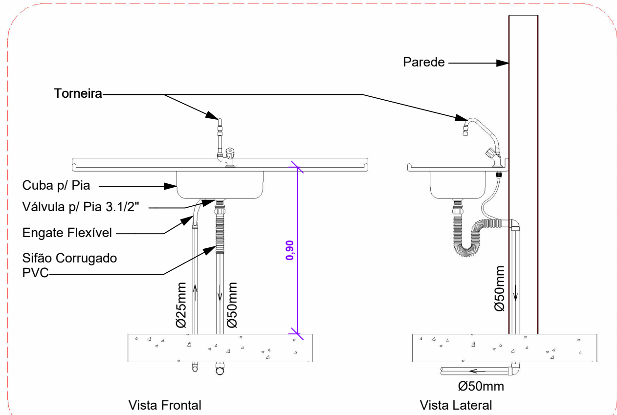
12 - Detalhe - Pia de Cozinha 1 : 20
