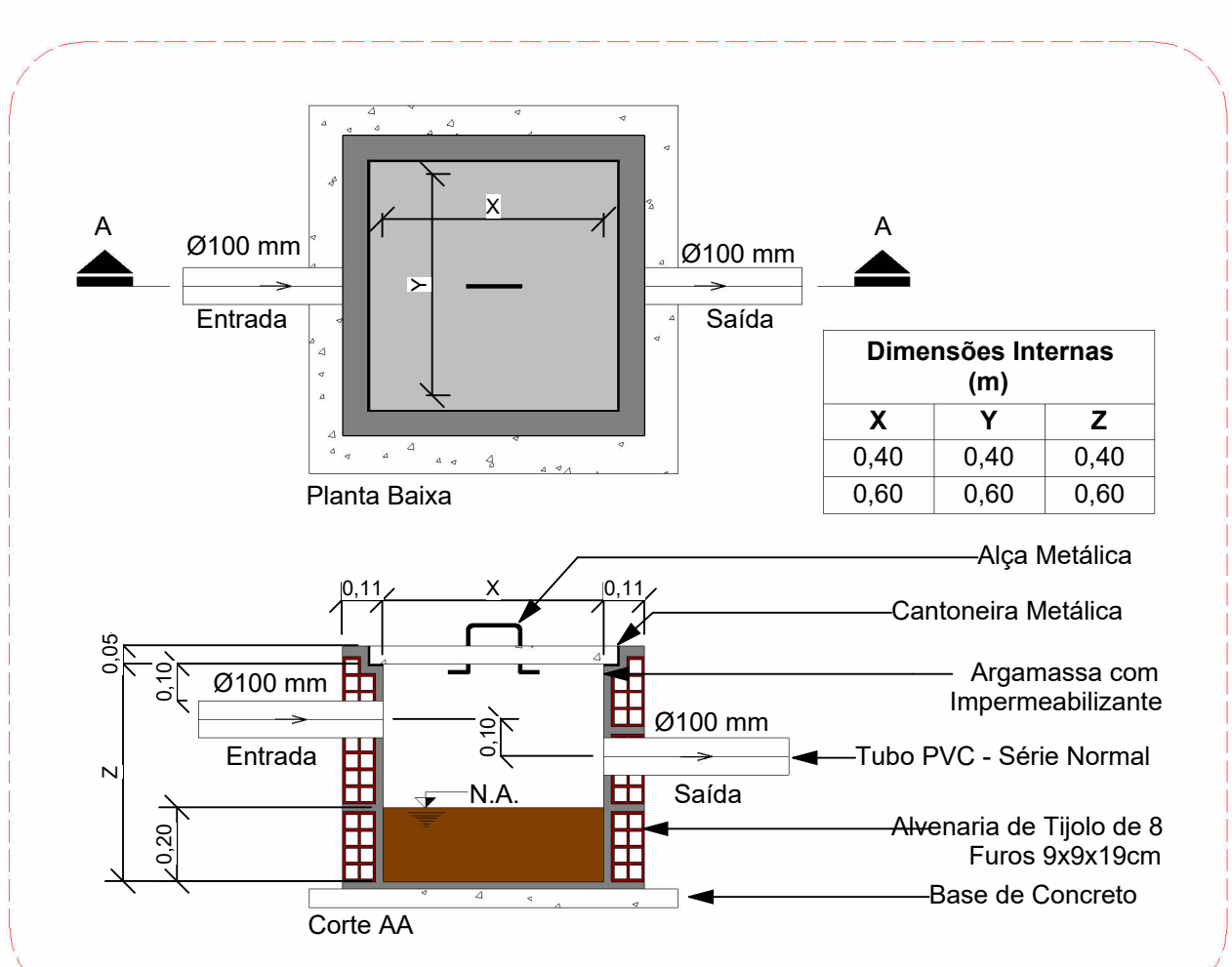
11 - Detalhe - Caixa de Areia 1 : 20
