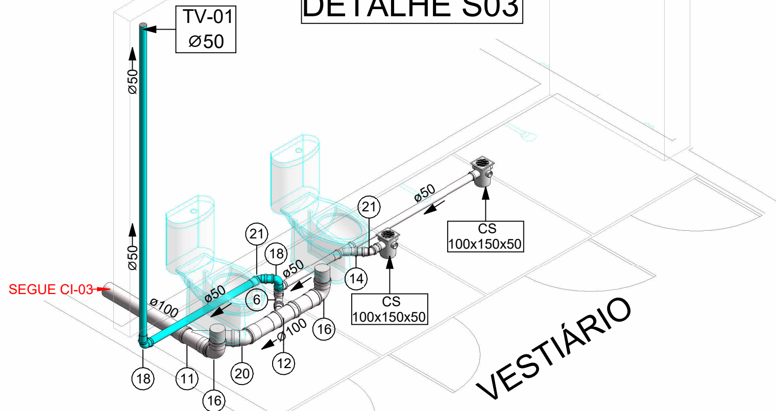
ISO DETALHE S03
