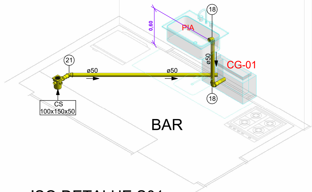
ISO DETALHE S01
