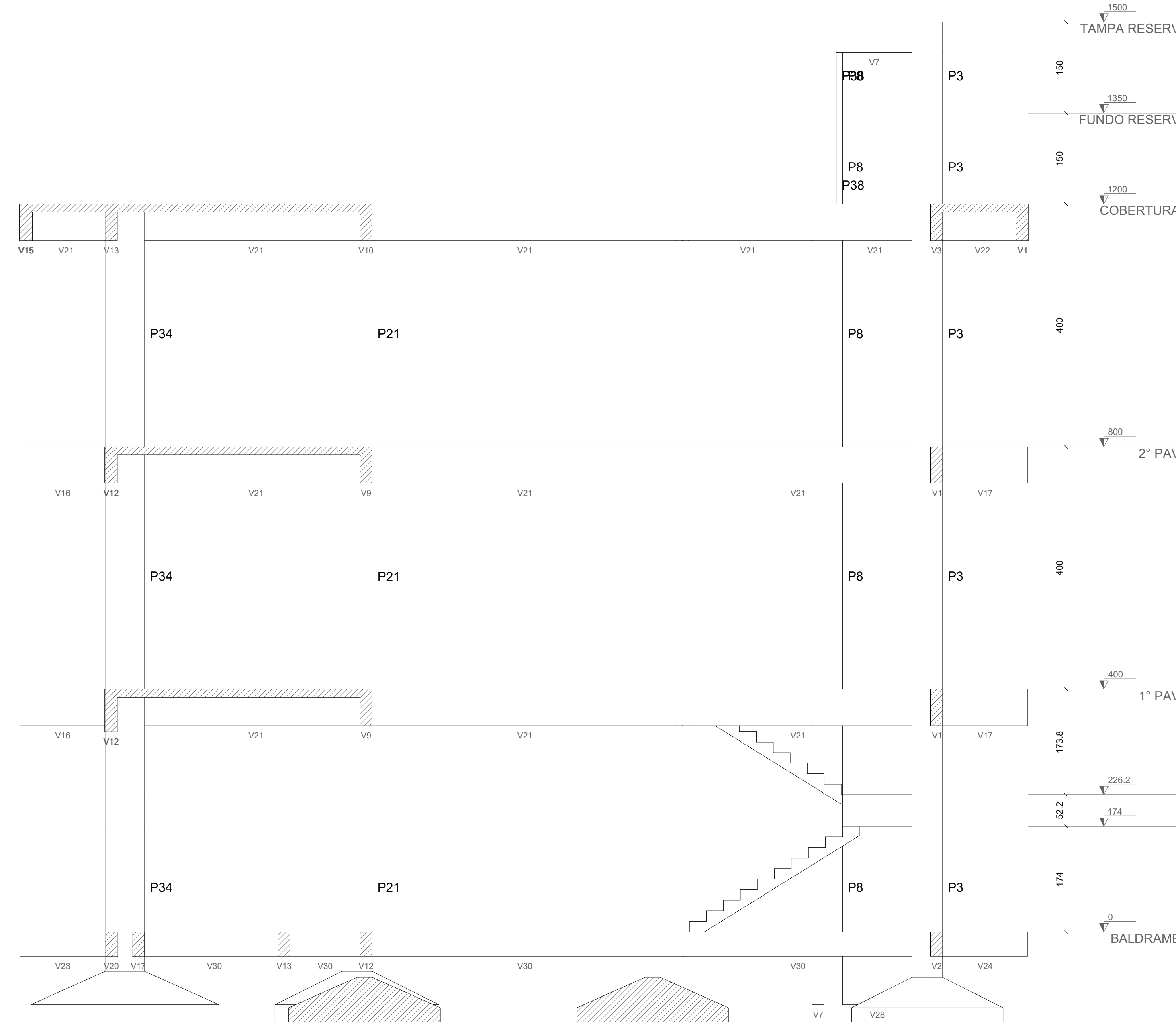
Corte B-B escala 1:50
